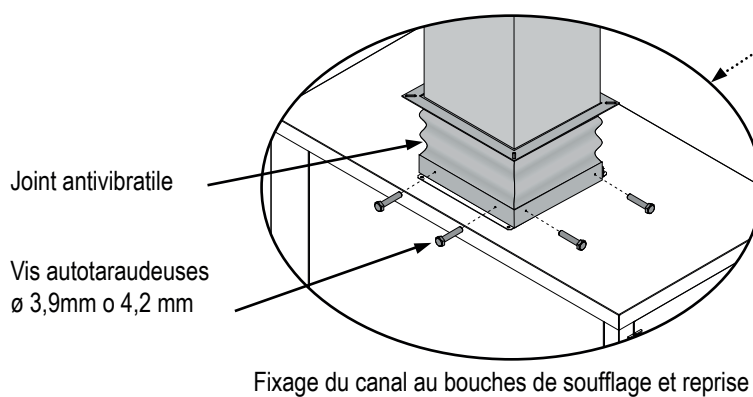
ASRI Soufflage horizontal droit
