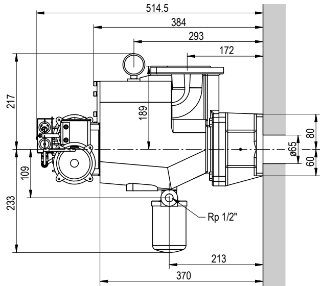
VUE LATÉRALE
