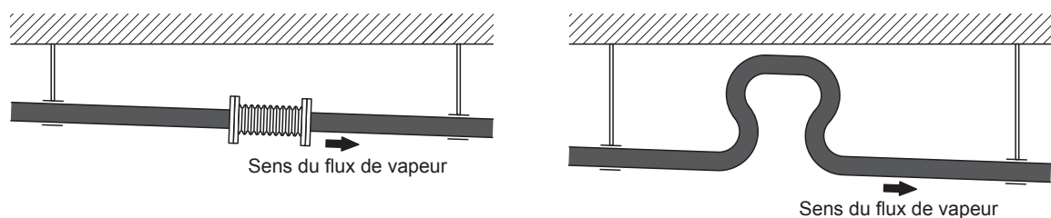
Fig. 43 : Suspensions/compensateurs
