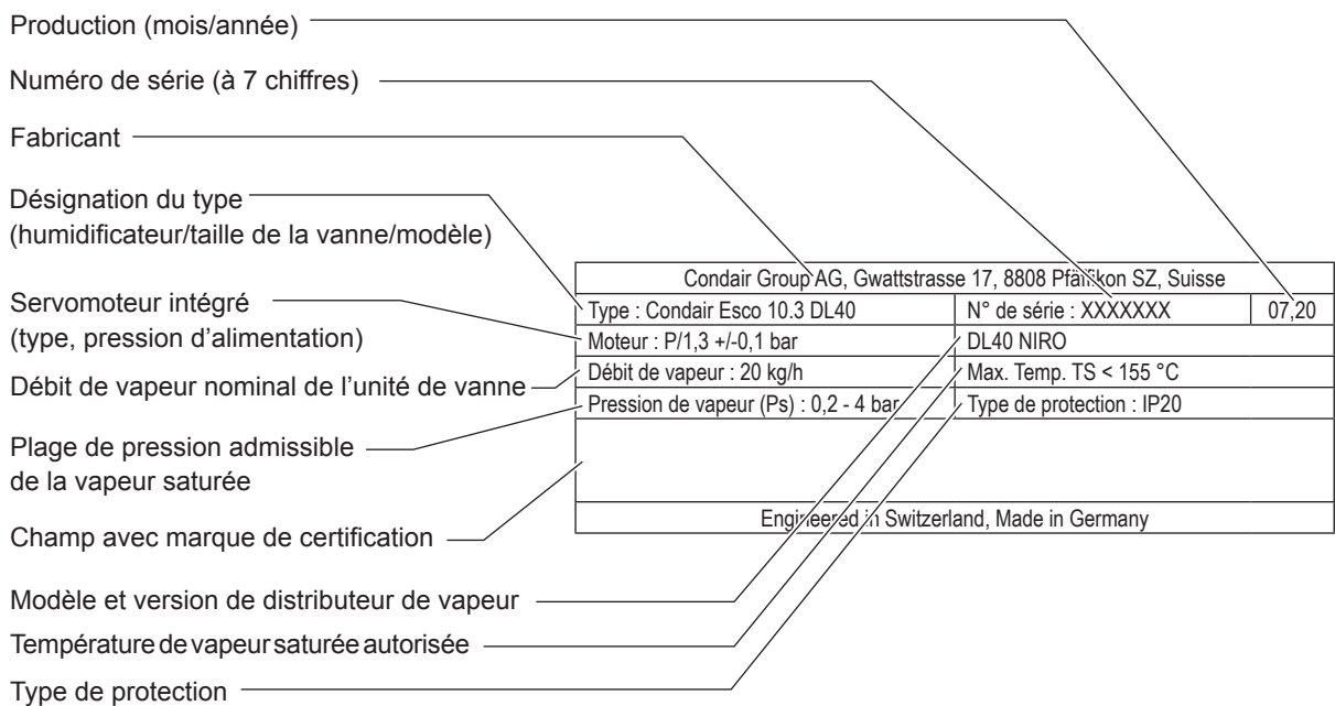
Fig. 9 : Exemple de plaque signalétique pour Condair Esco avec servomoteur pneumatique
