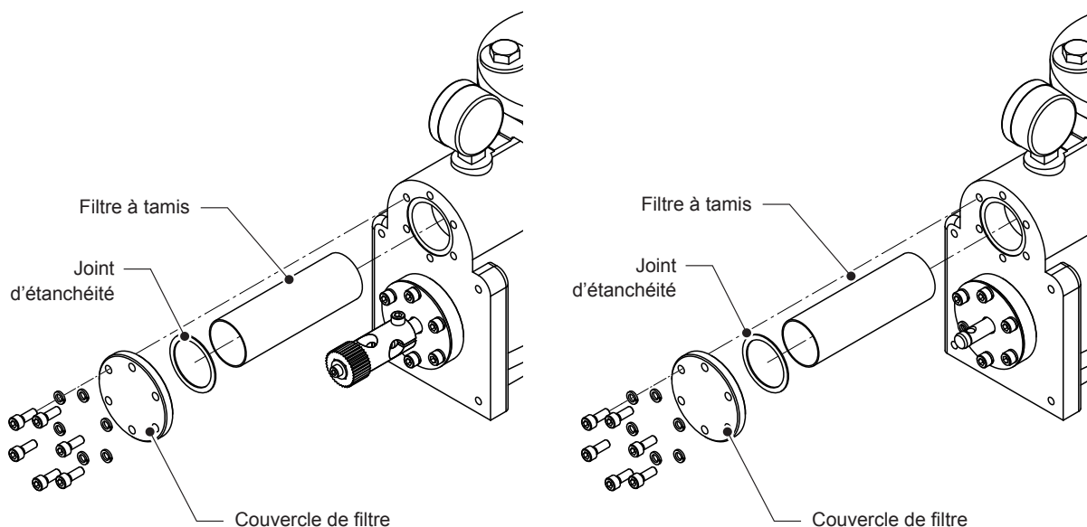
Fig. 56 : Démontez le filtre à tamis
