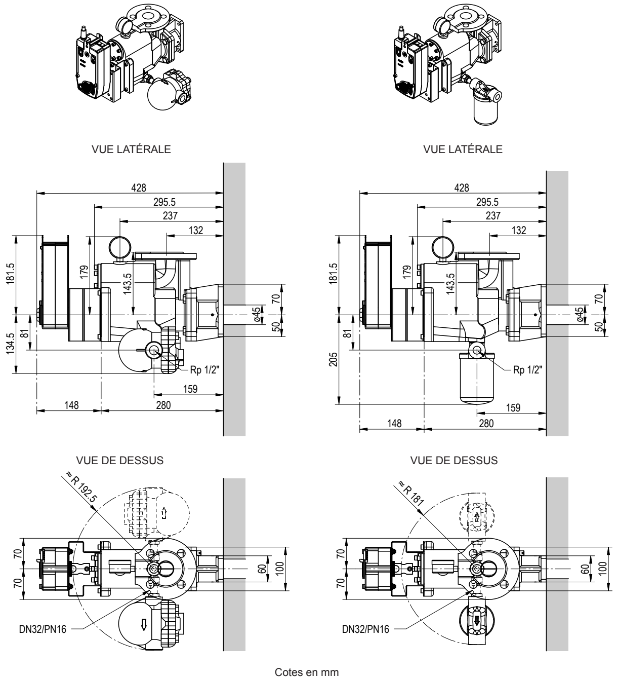
Fig. 60 : Schéma coté Esco 10 fonte ductile avec purgeur à flotteur sphérique avec servomoteur électrique CA150A-MP
