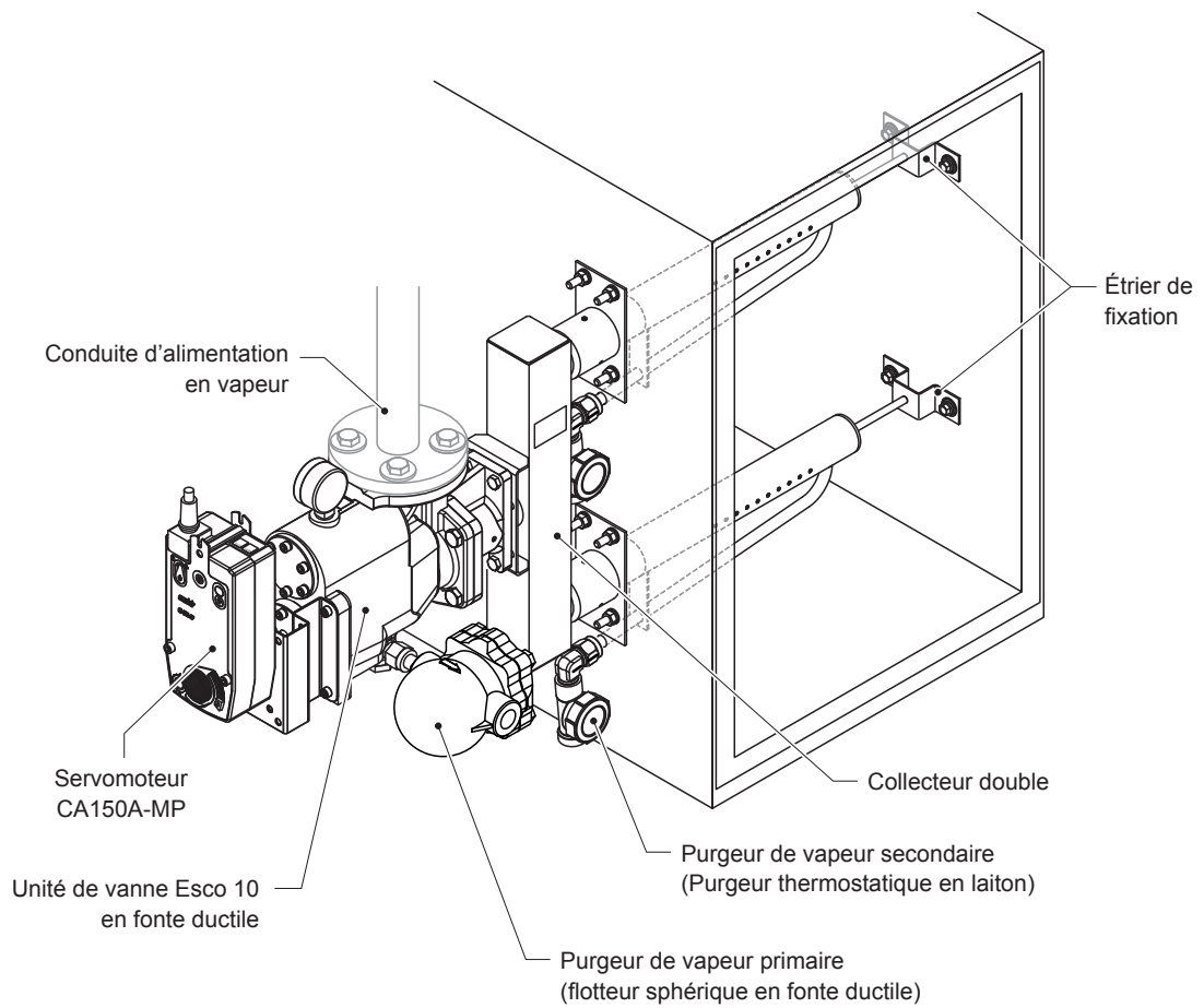
Fig. 2 : Aperçu d'installation Condair Esco 10 fonte ductile avec DL40 double collecteur
