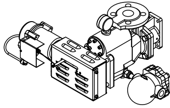
VUE LATÉRALE
