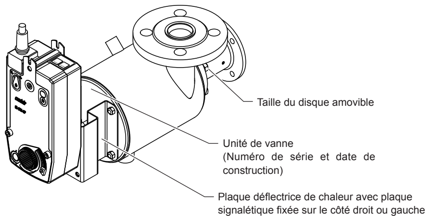
Fig. 7 : Positionnement de la plaque signalétique
