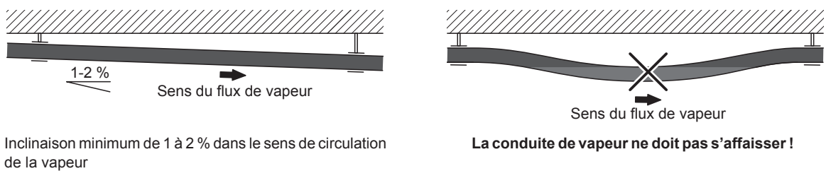
Fig. 42 : La pente dans le sens de circulation de la vapeur/la conduite de vapeur ne doit pas s'affaisser
