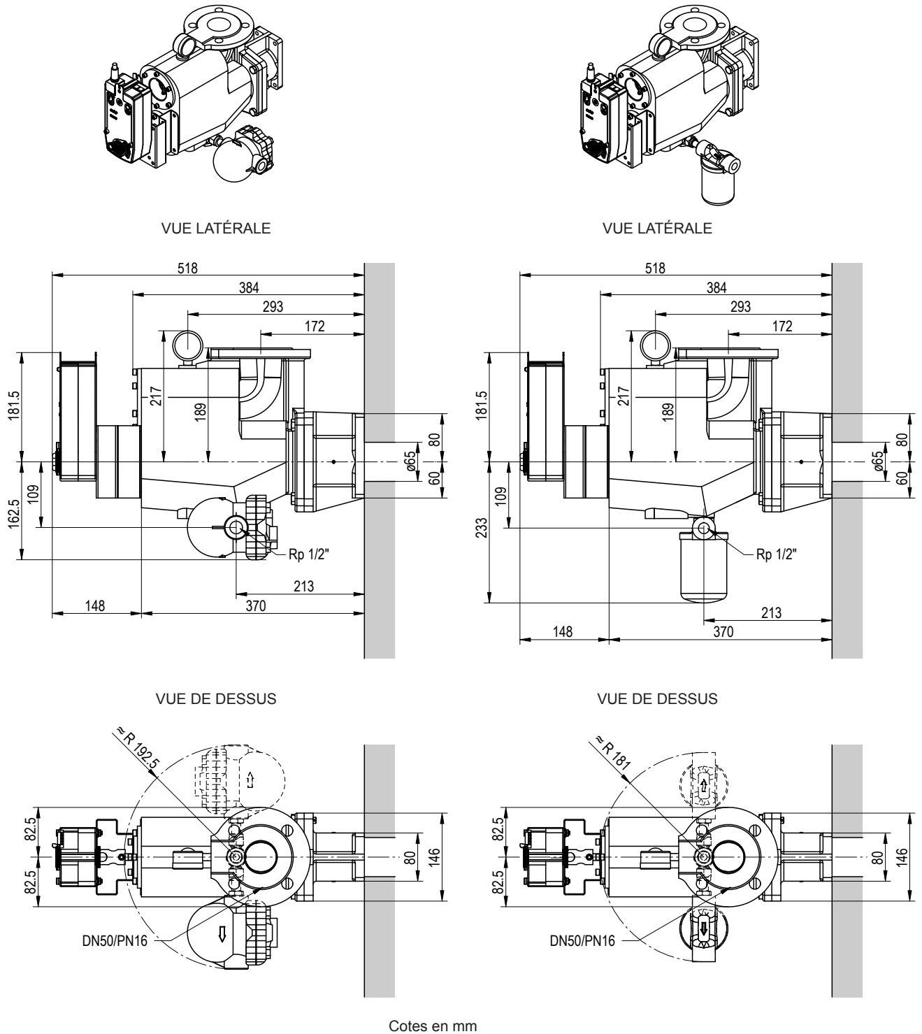
Fig. 68 : Schéma coté Esco 20 fonte ductile avec purgeur à flotteur sphérique avec servomoteur électrique CA150A-MP
