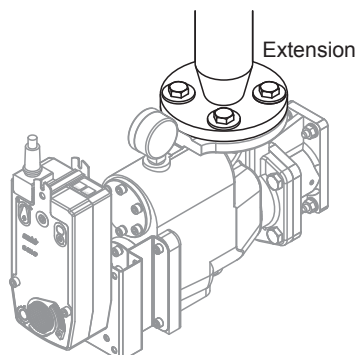
Fig. 37 : Extension de la conduite d'alimentation en vapeur
