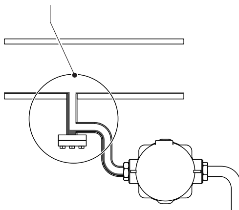
Fig. 40 : Drainage incorrect de condensats
