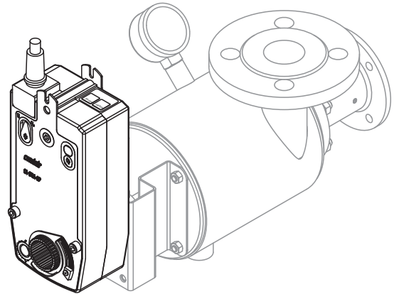
Condair Esco 10 en acier inoxydable avec servomoteur électrique CA150A-MP
