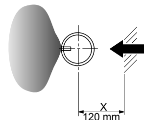
Fig. 27 : Gaine de ventilation/unité de traitement d'air avec DL40: distance aux obstacles en amont et en aval
