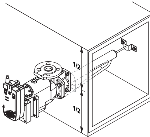
Fig. 23 : Version avec un tube à vapeur simple
