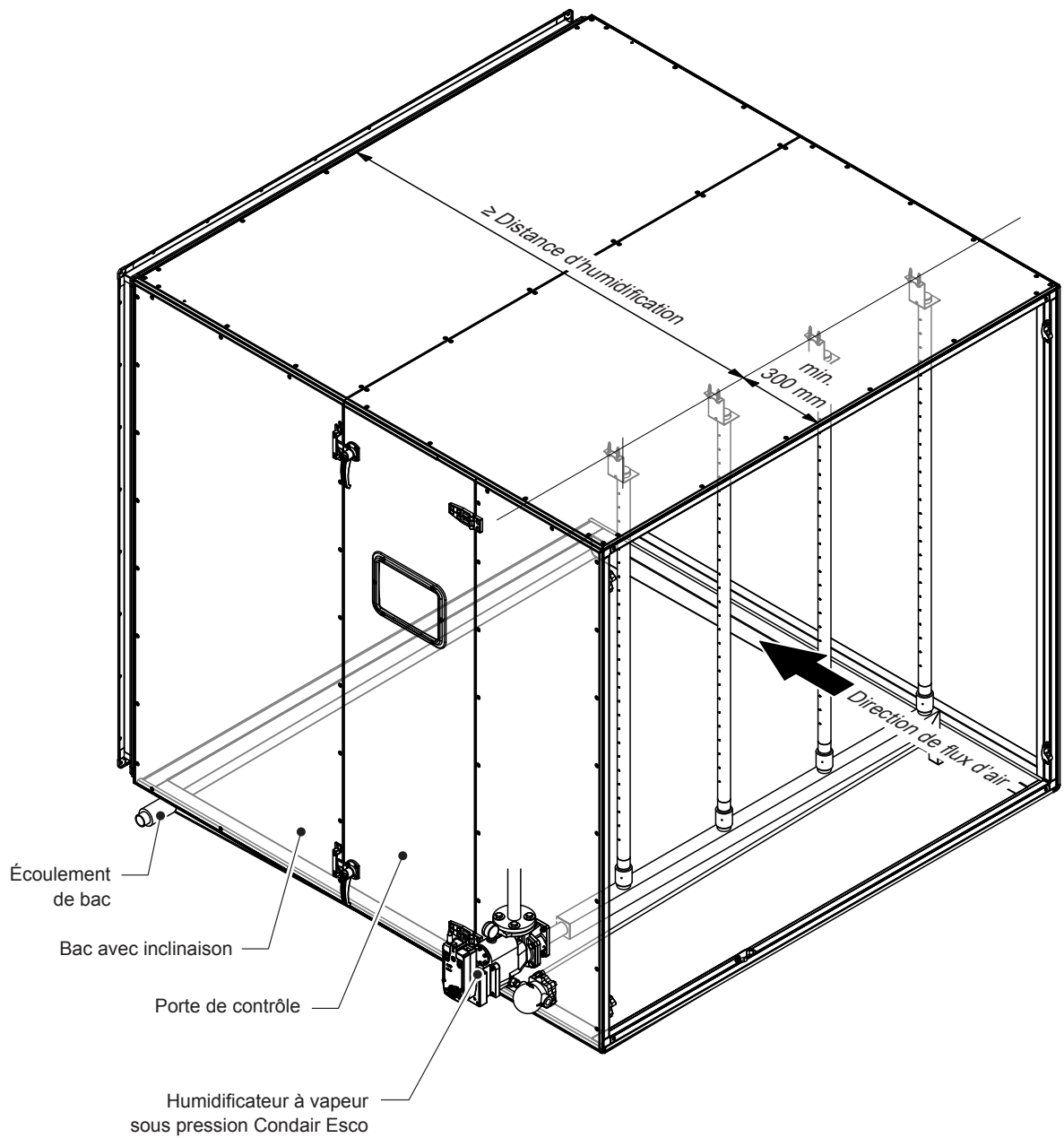
Fig. 28 : Gaine de ventilation/unité de traitement d'air avec DR73: distance aux obstacles en amont et en aval
