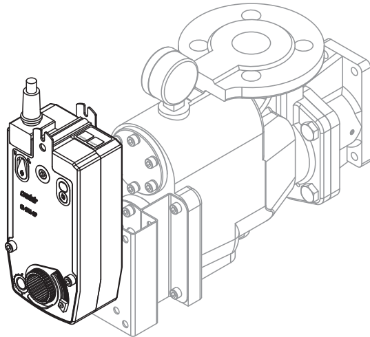
Fig. 16 : Servomoteur CA150A-MP
