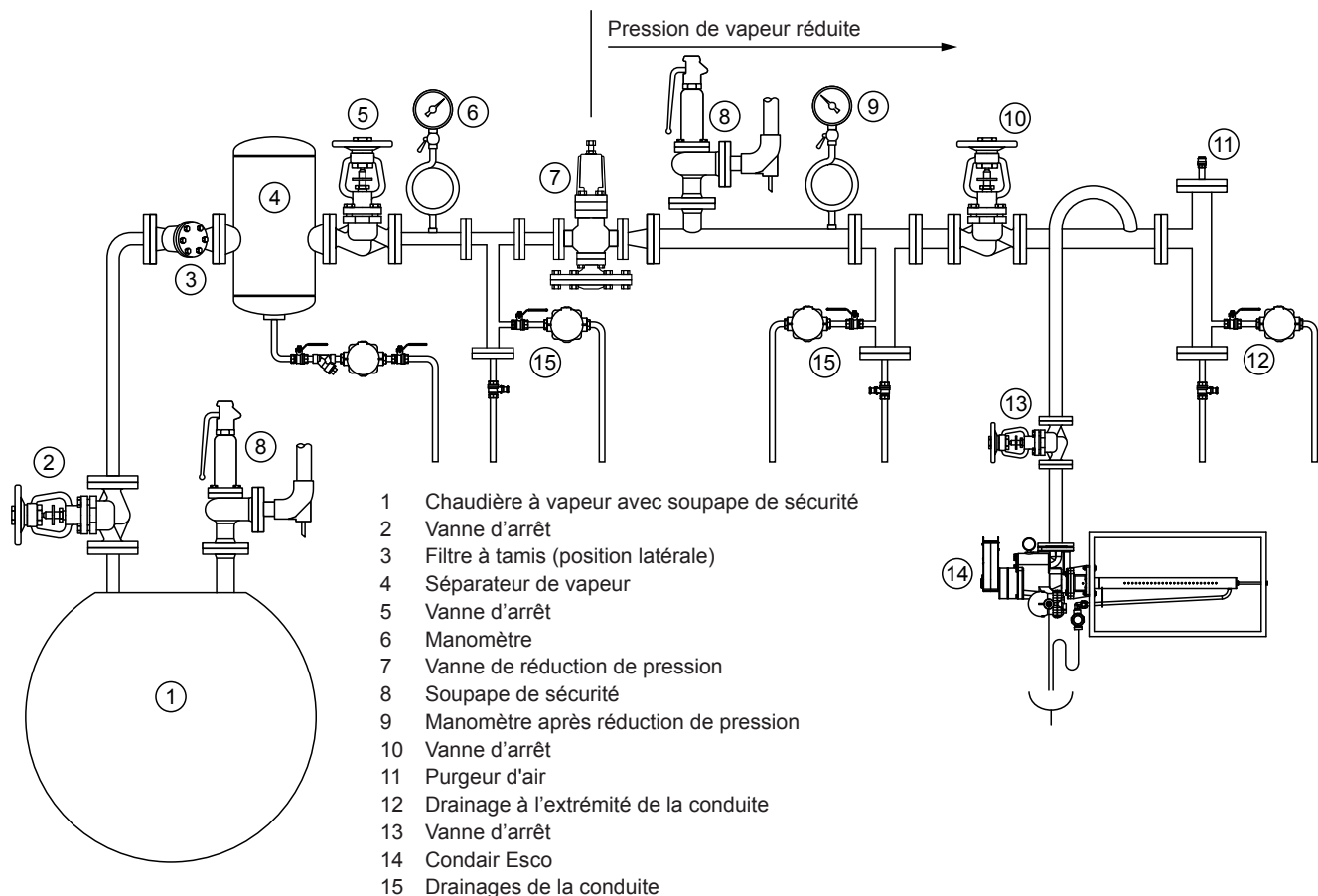
Fig. 35 : Schéma de principe du réseau de vapeur
