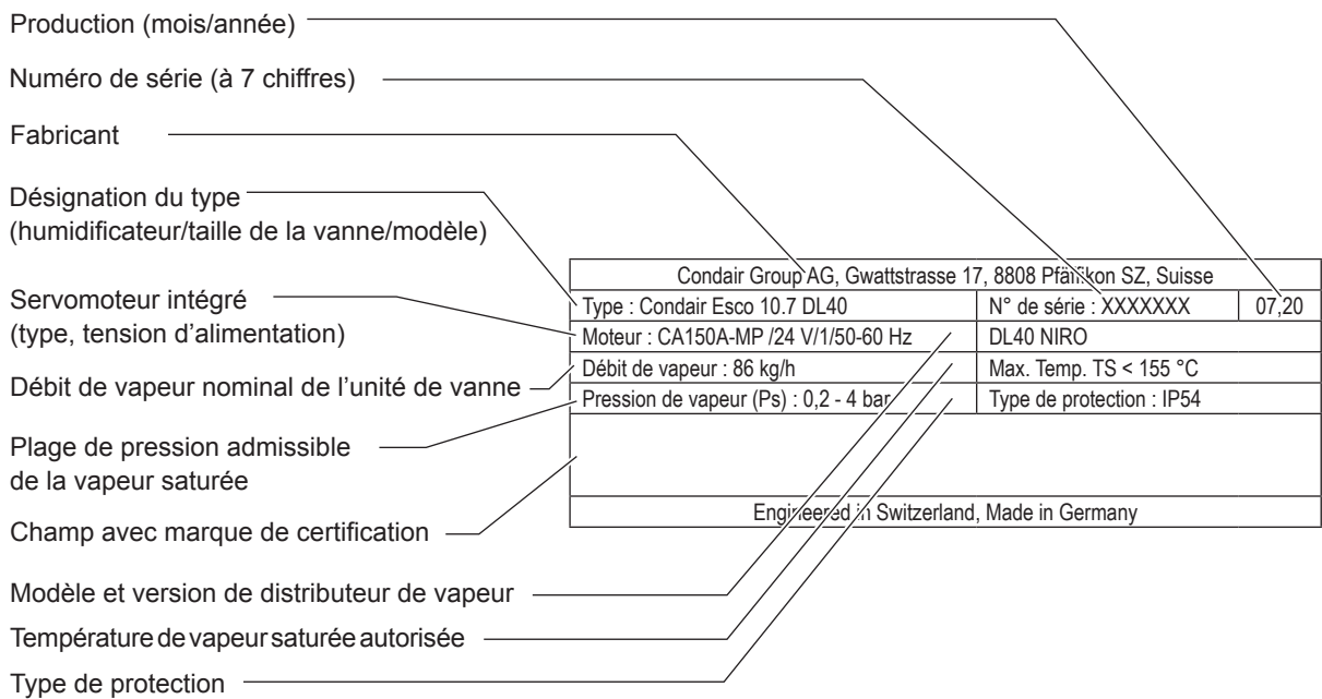
Fig. 8 : Exemple de plaque signalétique pour Condair Esco avec servomoteur électrique CA150A-MP
