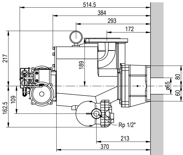
VUE LATÉRALE
