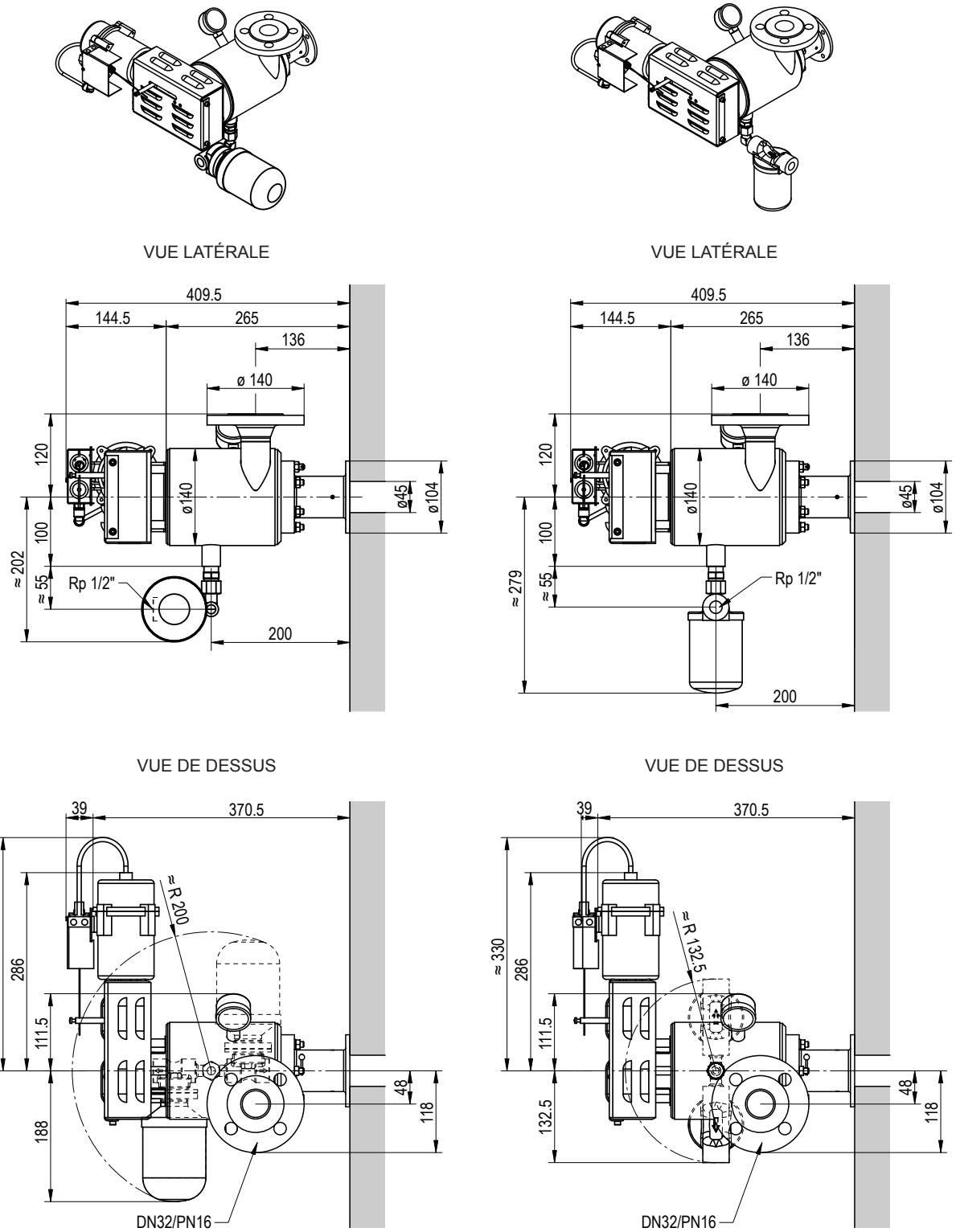
Fig. 66 : Schéma coté Esco 10 acier inoxydable avec purgeur à flotteur sphérique avec servomoteur pneumatique Sauter AK41
