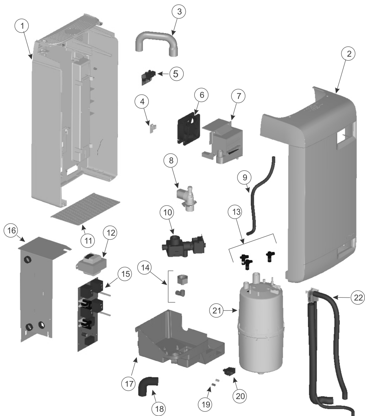
Figure 37: Vue éclatée de l'humidificateur RH2+
