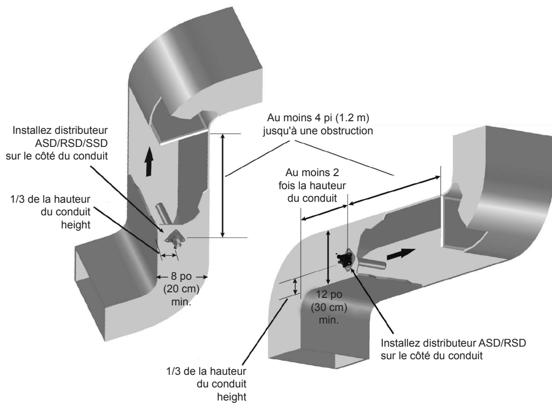
Figure 8: Installation du distributeur RSD10, ASD10 et SSD (RH2+ à conduit)
