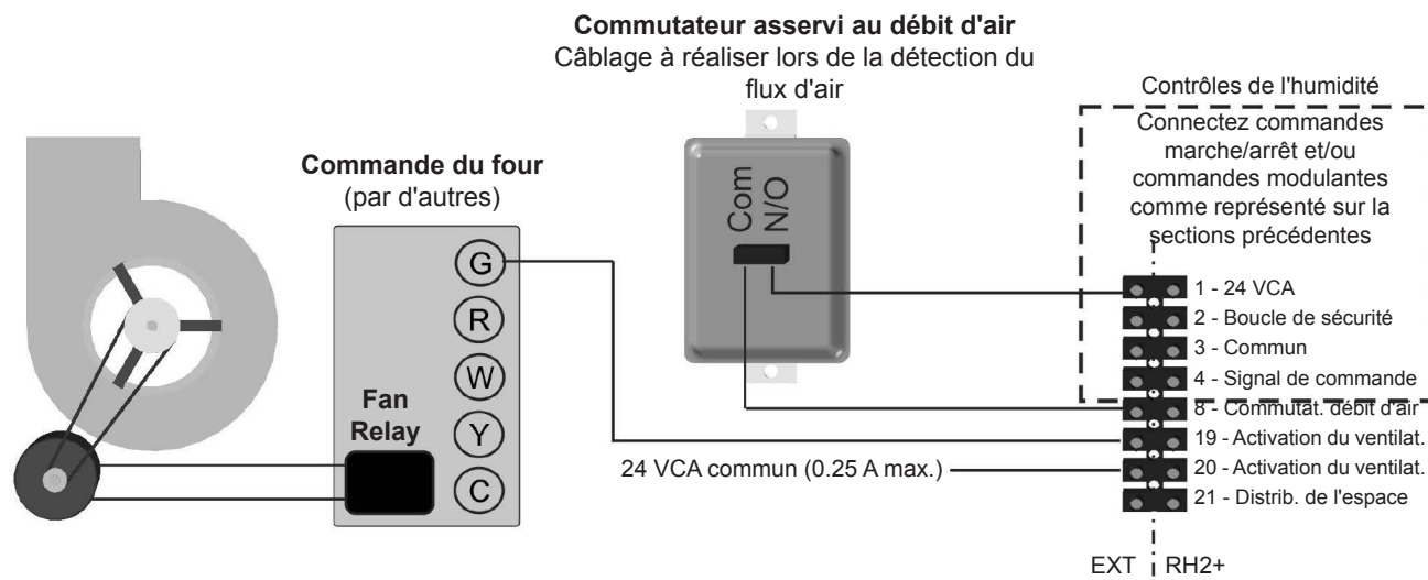
Figure 22: Câblage d'activation du ventilateur RH2+
