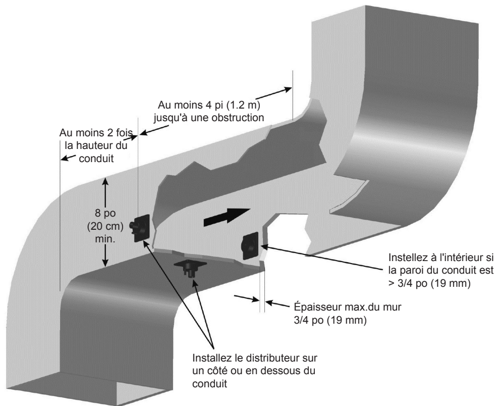
Figure 7: Installation du distributeur de buse (RH2+ à conduit)
