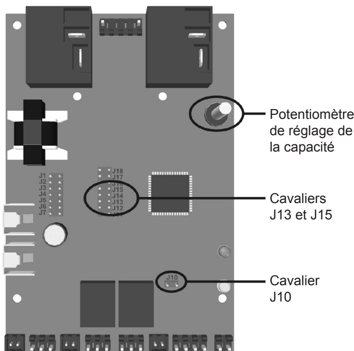
Figure 31: Cavaliers du panneau de commande RH2+
