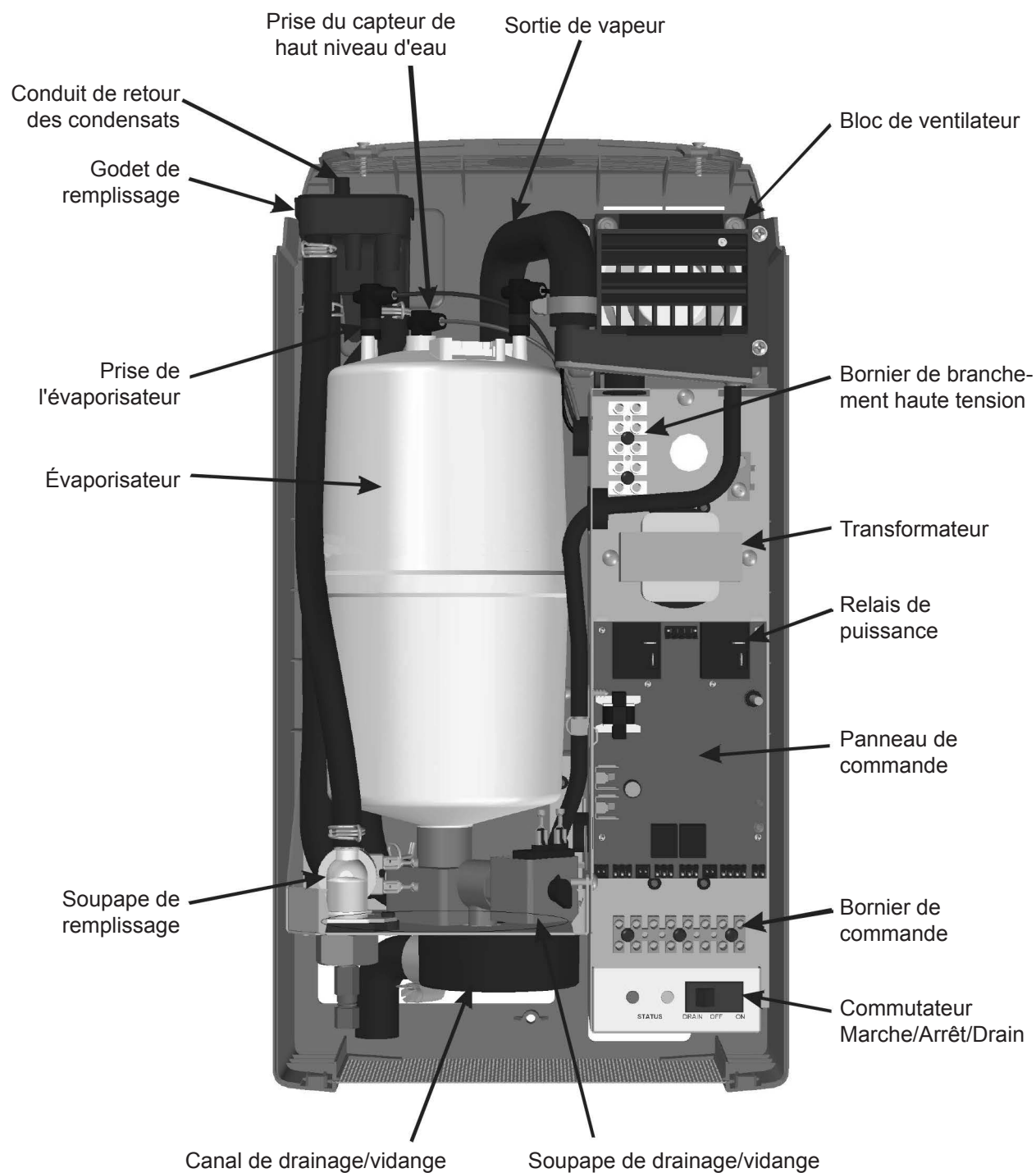
Figure 28: Composants de l'humidificateur RH2+
