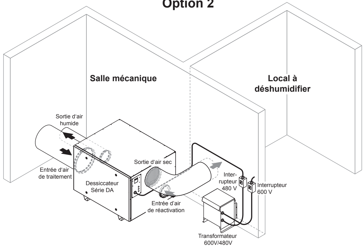
Fig. 22: Installation du dessiccateur série DA et du transformateur dans la salle mécanique
