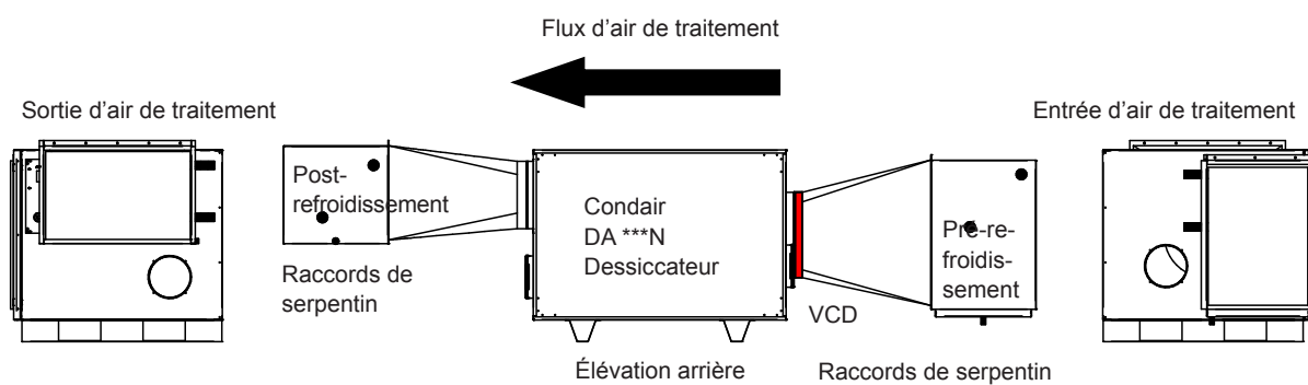
Fig. 13: Disposition d'installation des modules de refroidissement avec le dessiccateur DA
