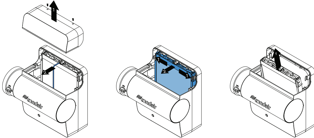
Figure 5 - Remplacement de l'élément en céramique
