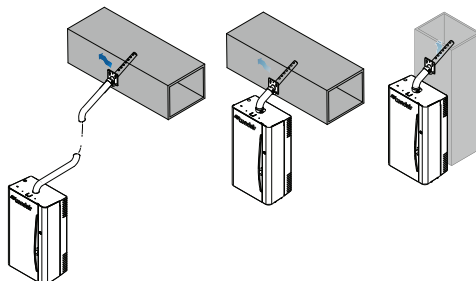
Figure 2 - Installations de l'humidificateur RH sur conduite et à distance
