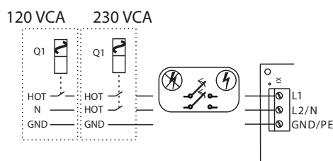
Figure 14 - Connexion haute tension et déconnexion externe
