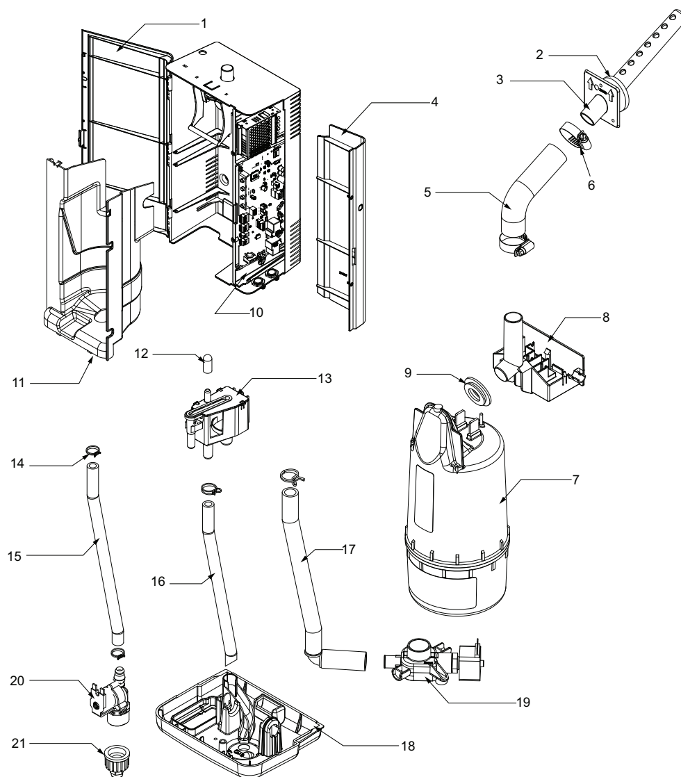
Figure 1 - Composants de l'humidificateur RH
