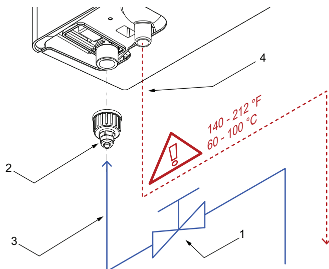
Figure 13 - Raccordement de l'alimentation en eau et du système de vidange
