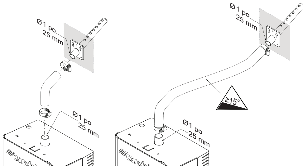
Figure 11 - Installation de la conduite et du distributeur de vapeur
