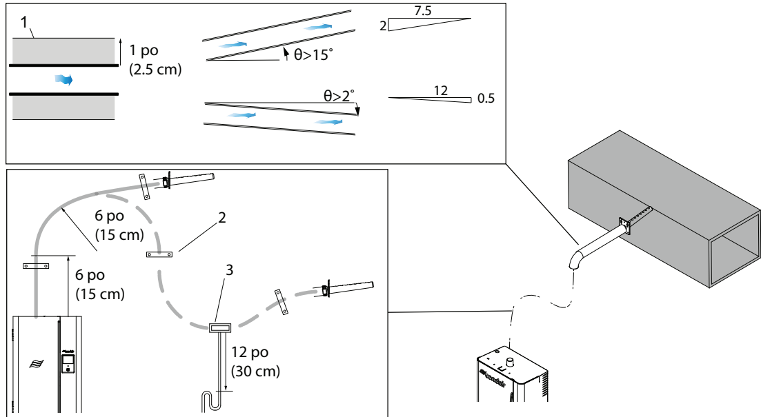
Figure 10 - Installation montée à distance avec distributeur de vapeur (vue horizontale)
