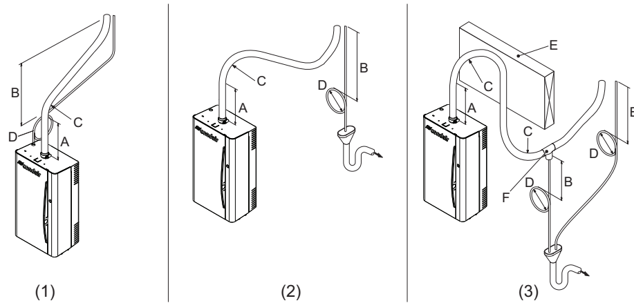
Figure 7 - Considérations relatives à la conduite de vapeur et de condensat (installations distantes)
