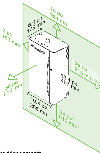
Figure 8 - Emplacement et dégagements
