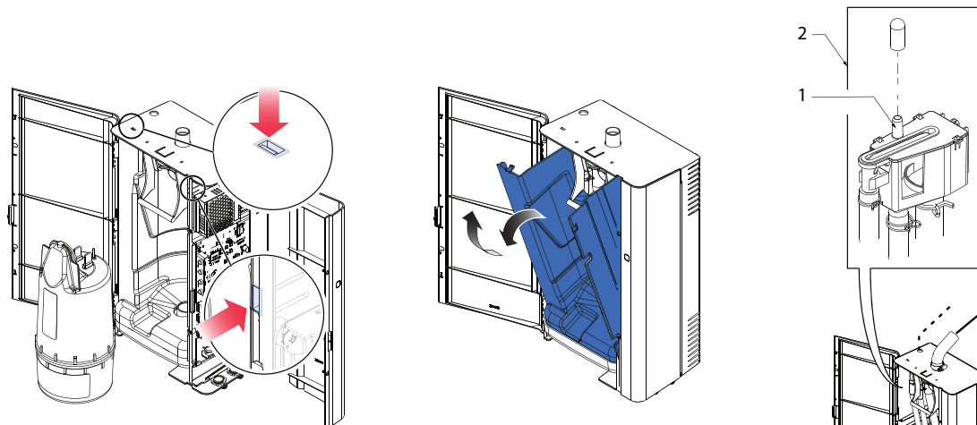
Figure 12 - Dépose du cache tuyauterie et installation de la conduite de retour du condensat
