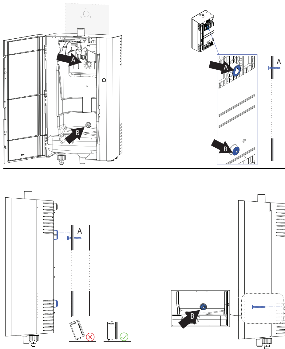
Figure 9 - Montage de l'humidificateur sur le mur (montant) ou la conduite
