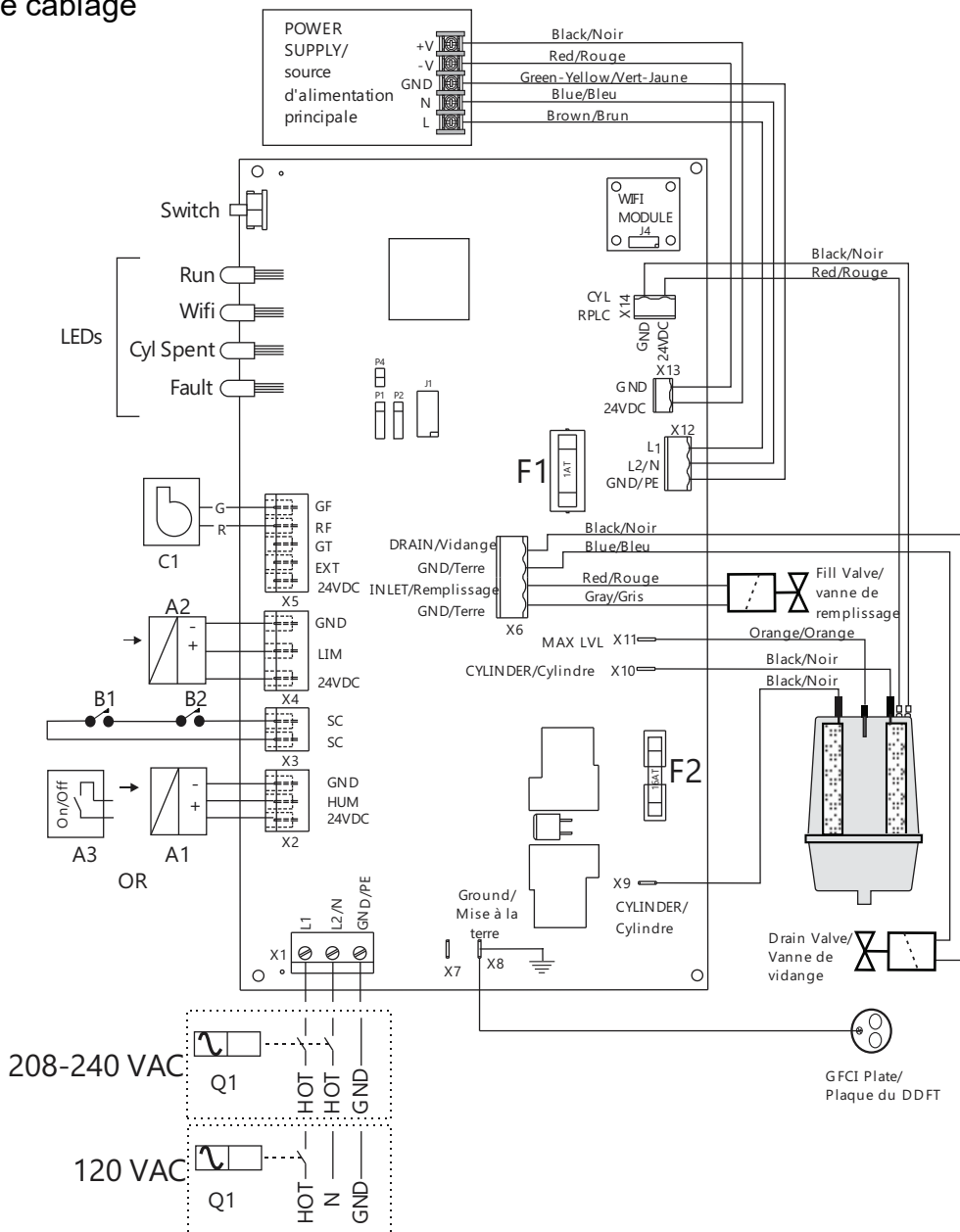
Figure 15 - Schéma de câblage
