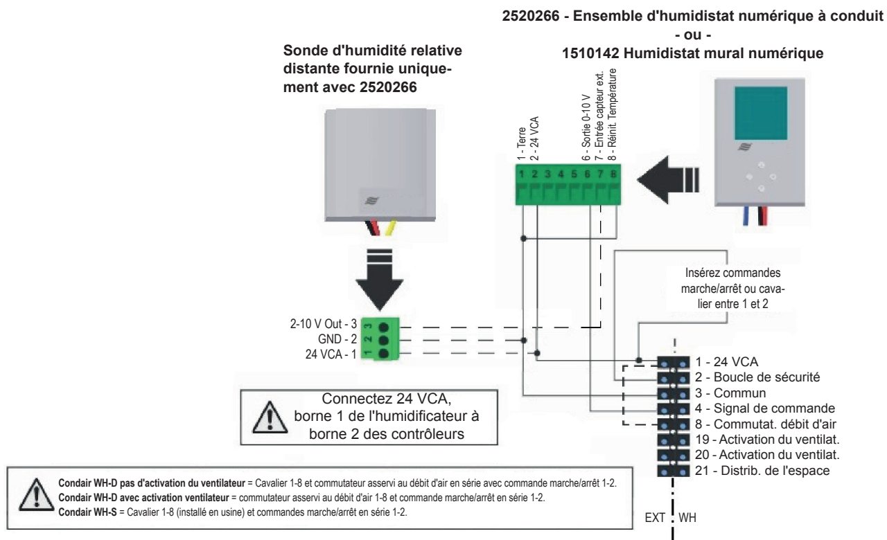
Figure 21: Câblage des commandes à modulation
