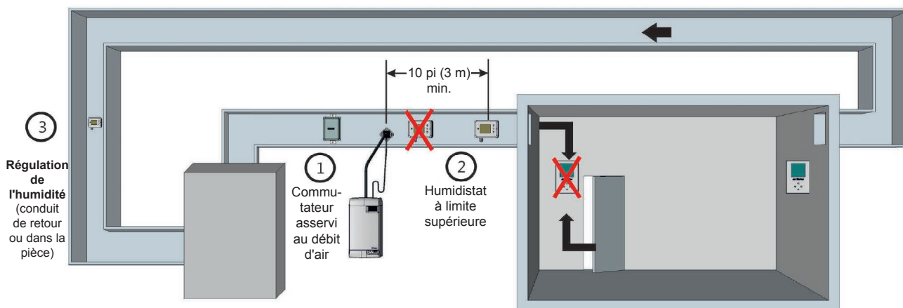
Figure 16: Emplacement des commandes (humidification des conduits)
